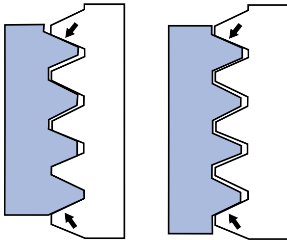
Angle error
